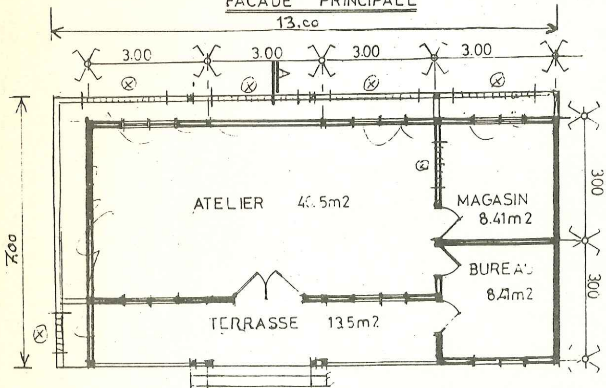
FACADE PRINCIPALE
