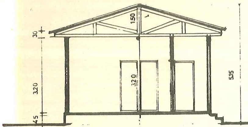
COUPE AA
